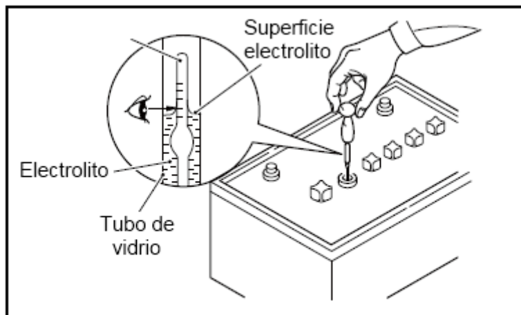
Fig. 8-26: Gravedad específica del electrolito de batería Revisión
