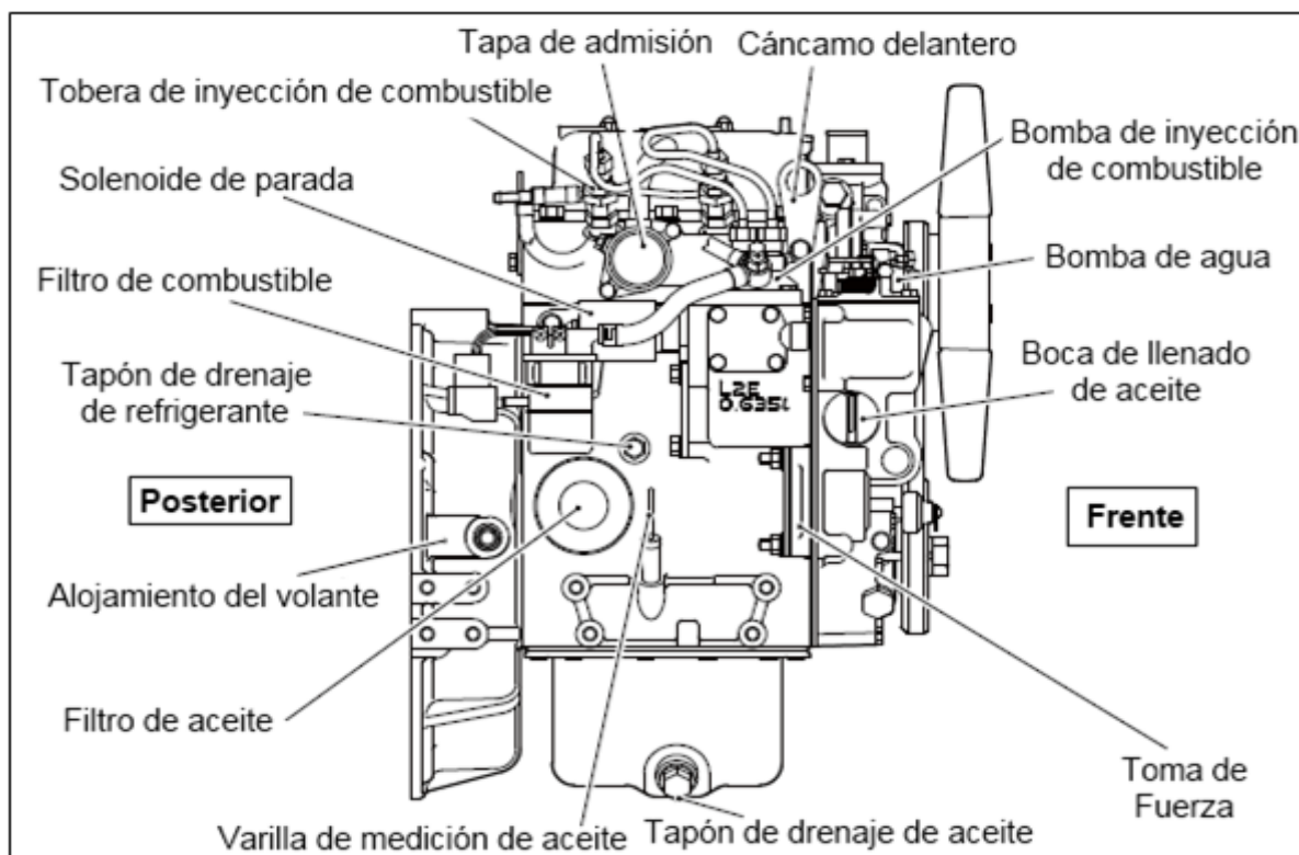
Fig. 2-2: Motor, vista derecha
