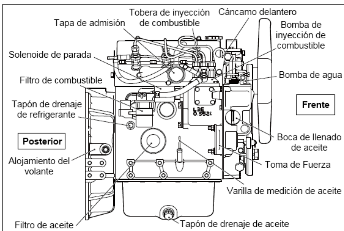
Fig. 2-4: Motor, vista derecha
