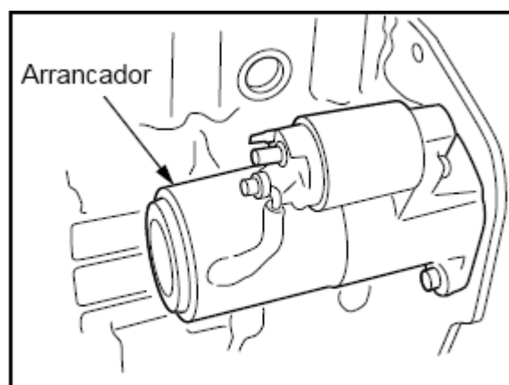
Fig. 8-27: Arrancador - Inspección
