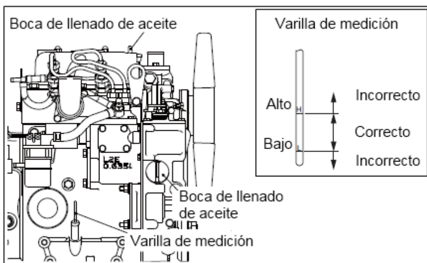
Fig. 8-12: Aceite de motor - Llenado
