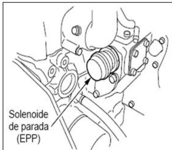
Fig. 2-10: Solenoide de parada
