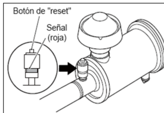
Fig. 2-13: Indicador del filtro de aire
