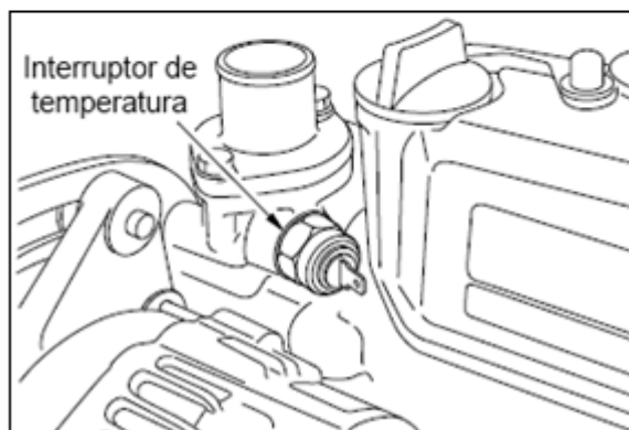
Fig. 2-12: Interruptor de temperatura
