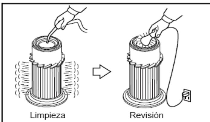
Fig. 8-23: Elemento del filtro de aire Inspección y Limpieza
