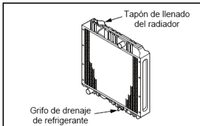
Fig. 8-16: Grifo de drenaje de refrigerante (radiador)
