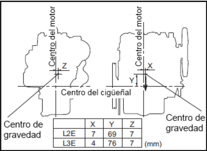
Fig. 10-2: Centro de gravedad del motor (especificación estándar)
