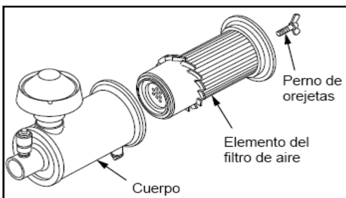
Fig. 8-22: Elemento del filtro de aire - Remoción
