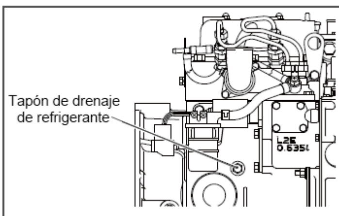
Fig. 8-17: Tapón de drenaje de refrigerante (motor)
