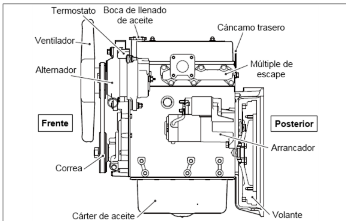
Fig. 2-3: Motor, vista izquierda
