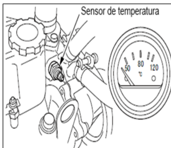
Fig. 2-7: Medidor de temperatura de agua y sensor de temperatura
