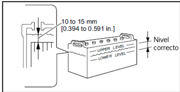
Fig. 8-25: Nivel de electrolito de la batería - Inspección
