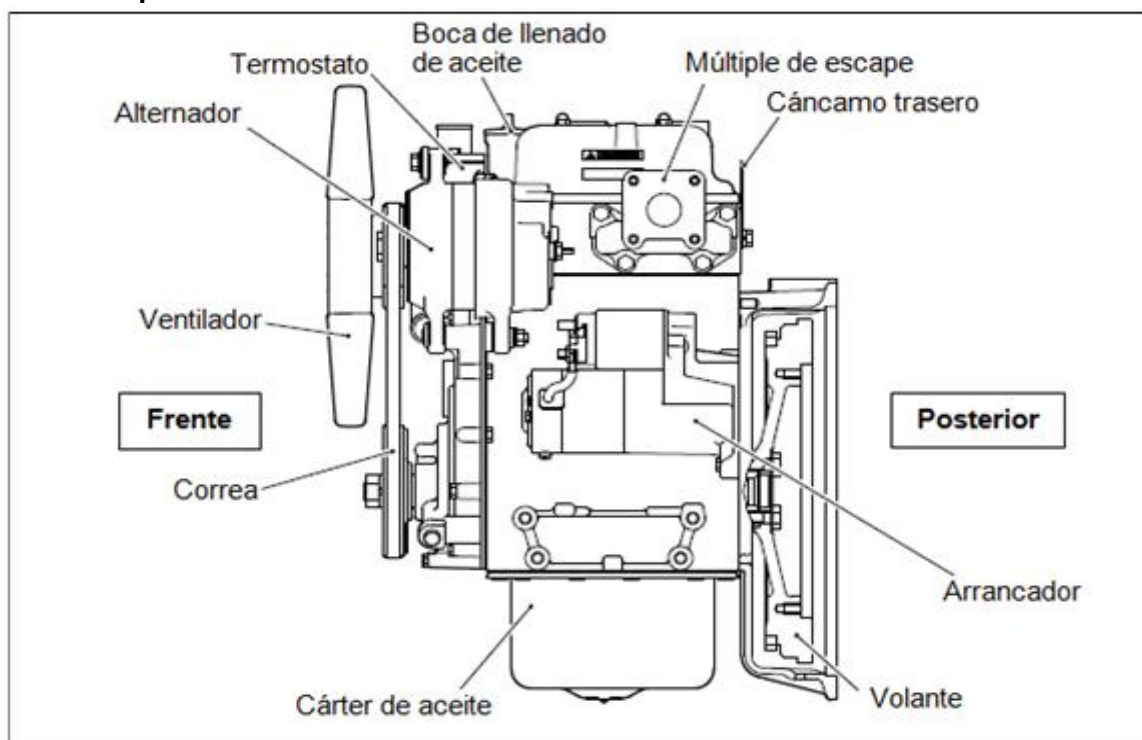
Fig. 2-1: Motor, vista izquierda
