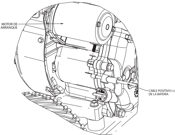
Figura 4 - Conexión de la batería
